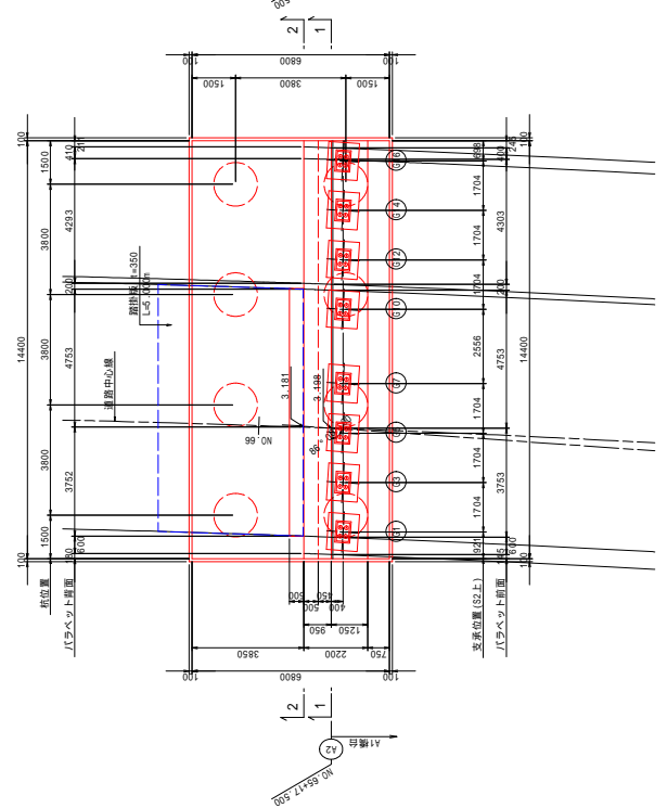
平面図
