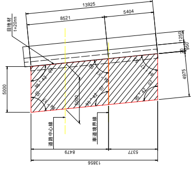
踏掛版
