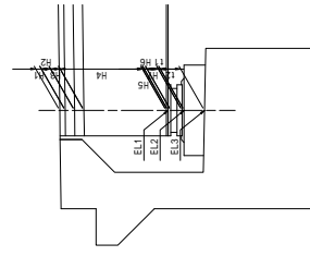
支承位置断面図
